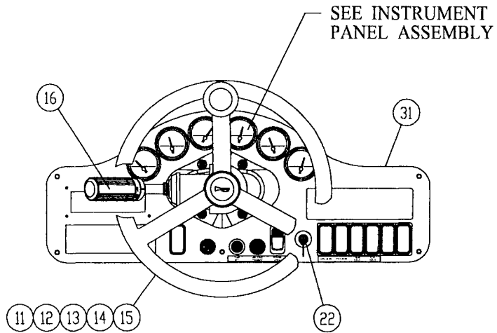
VIEW A-A
